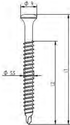
Eurofast EDS-B 5,5 x L
