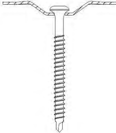
Eurofast EDS-B 4,8 x L
