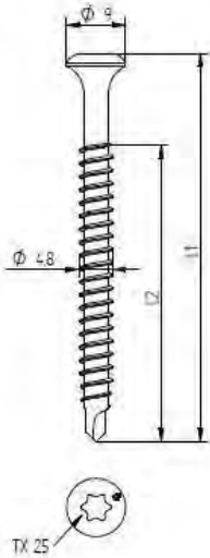
Eurofast EDS-B 4,8 x L
