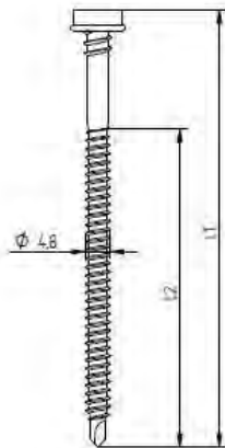
Eurofast EDS-BZT/BGT 4,8 x L
