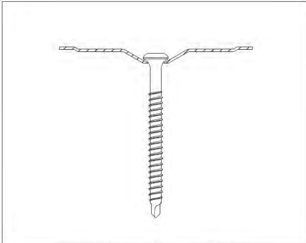
Eurofast EDS-SRB 4,8 x L
