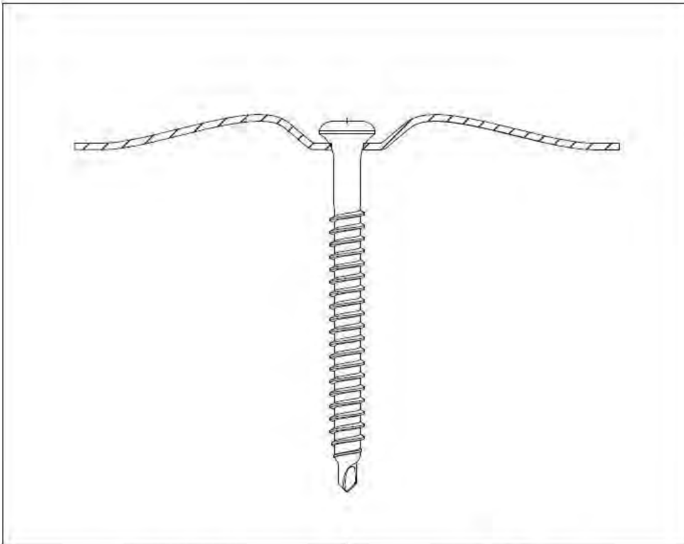
Eurofast EDS-B 5,5 x L
