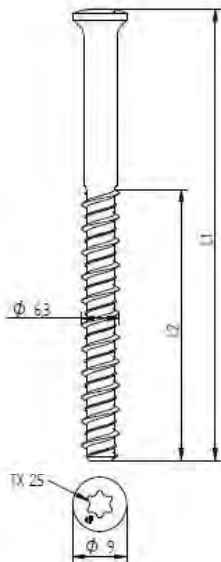
Eurofast EFR 6,3 x L
