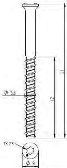
Eurofast EFR 6,3 x L
