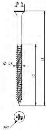
Eurofast EDS-S 4,8 x L
