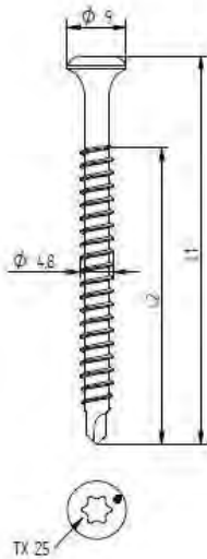
Eurofast EDS-SRB 4,8 x L
