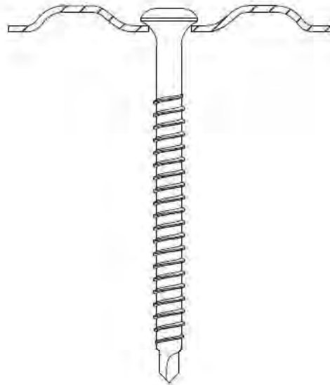
Eurofast EDS-SRB 4,8 x L
